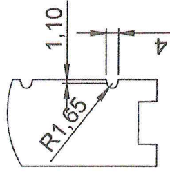
Detail B Maßstab 2 : 3
